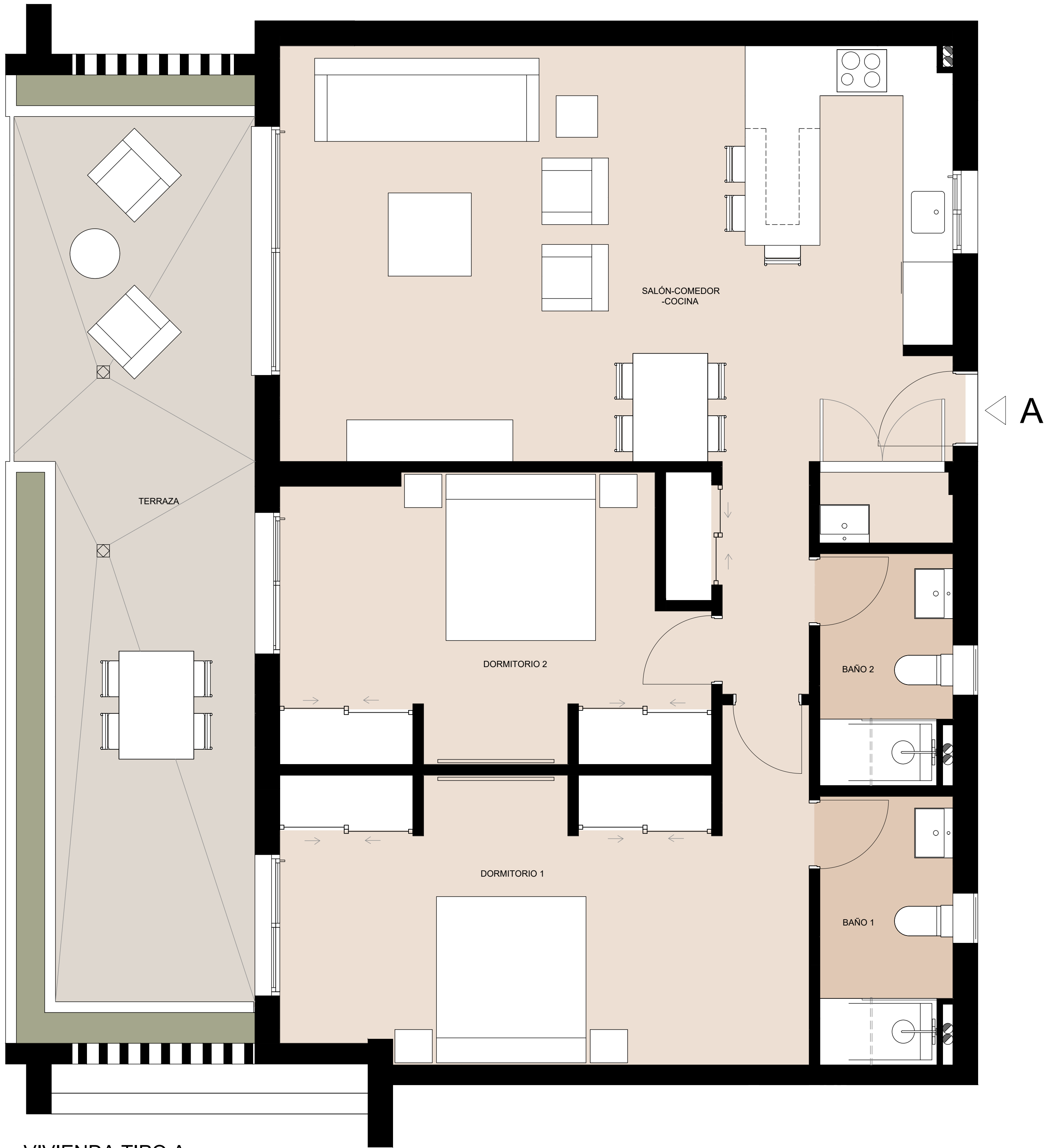
VIVIENDA TIPO A ESCALA: 1 : 50
