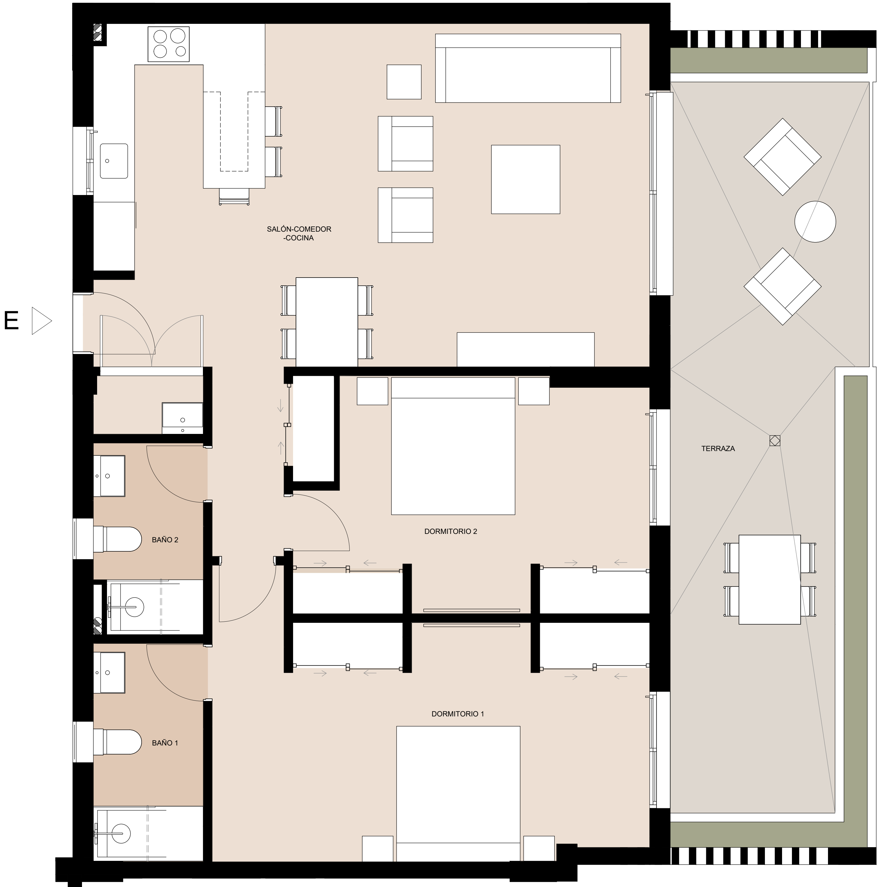
VIVIENDA TIPO E ESCALA: 1 : 50
