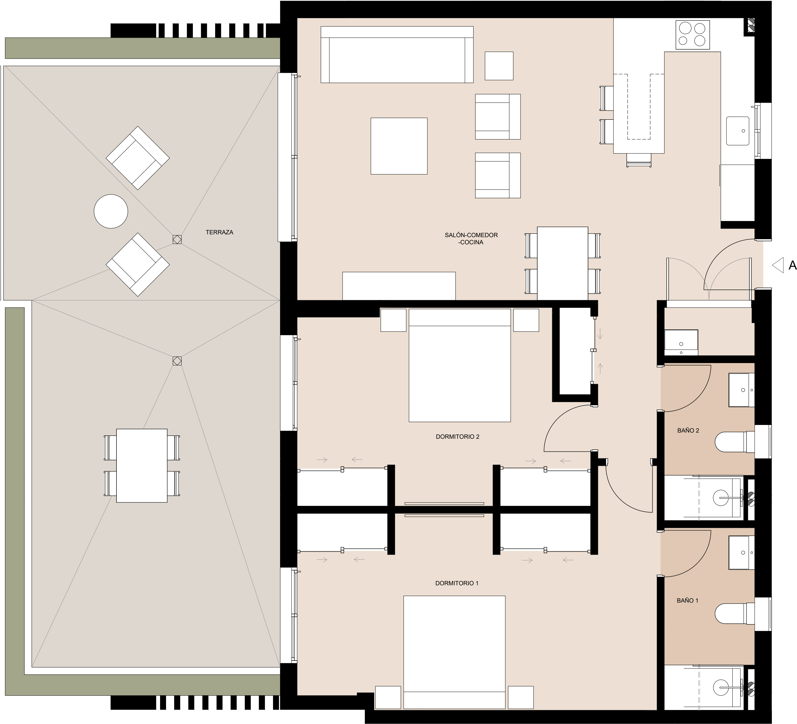
VIVIENDA TIPO A ESCALA: 1 : 50
