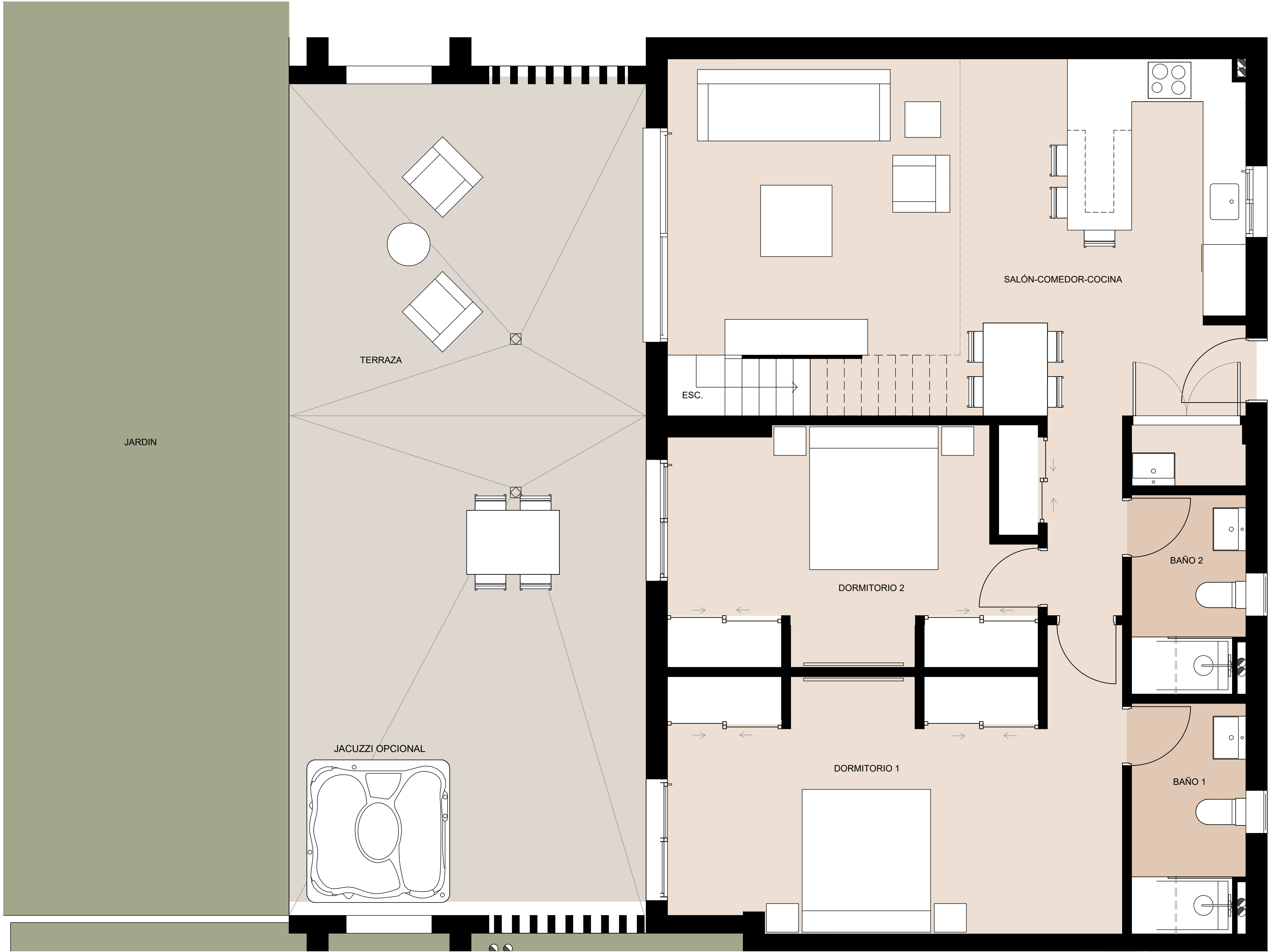
VIVIENDA TIPO A ESCALA:1 : 60
