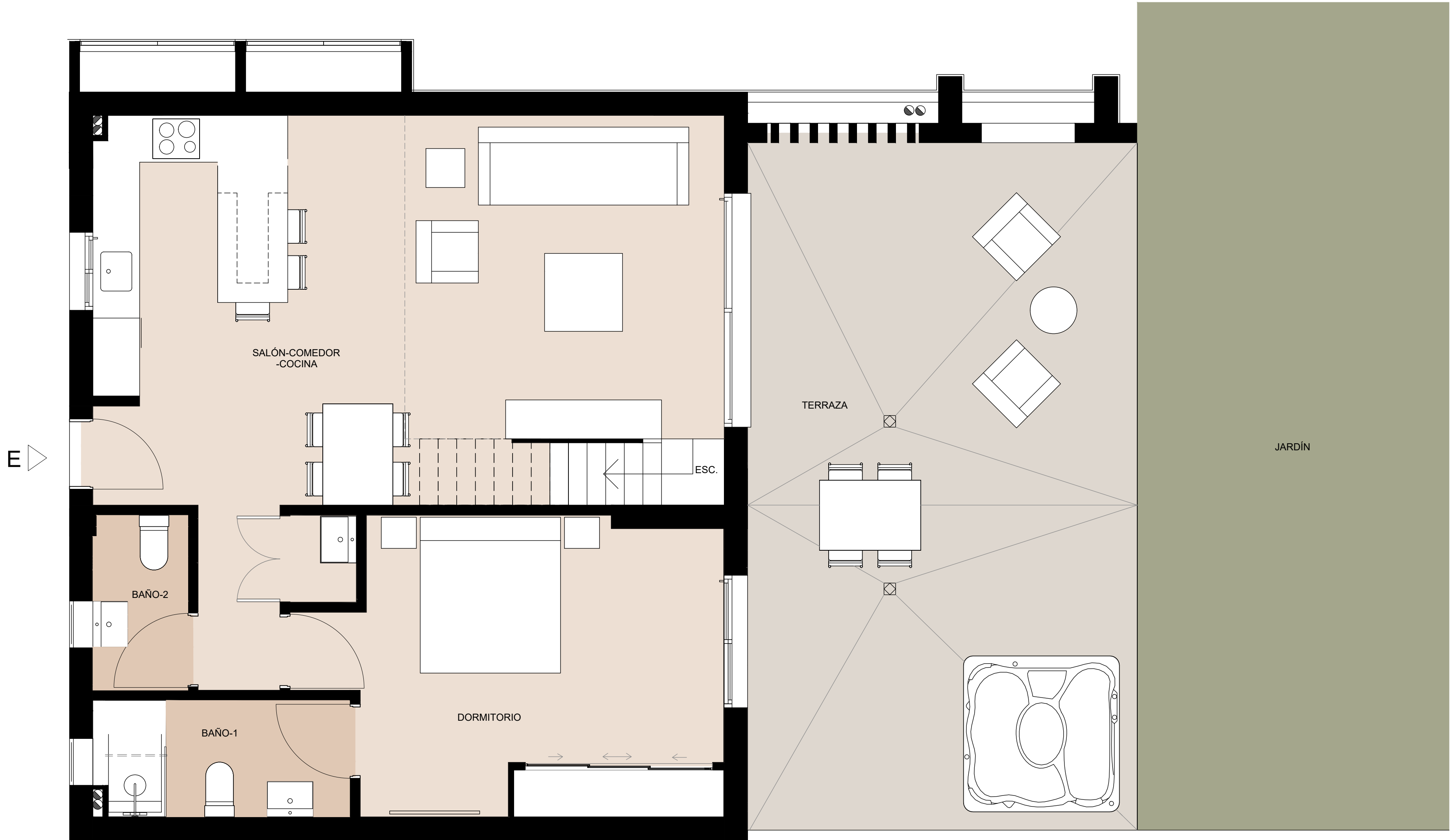
VIVIENDA TIPO E ESCALA:1 : 60
