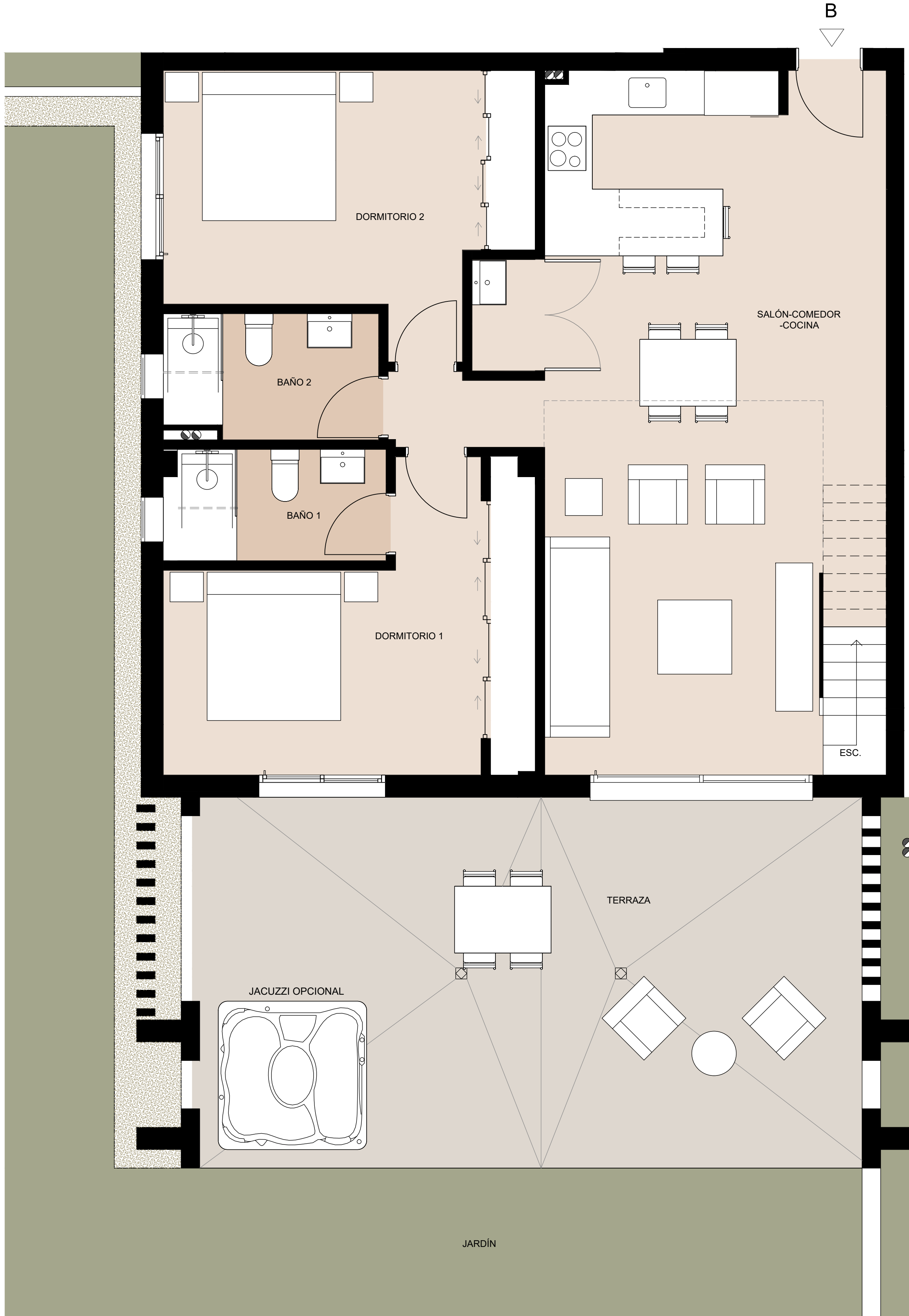
VIVIENDA TIPO B ESCALA:1 : 60
