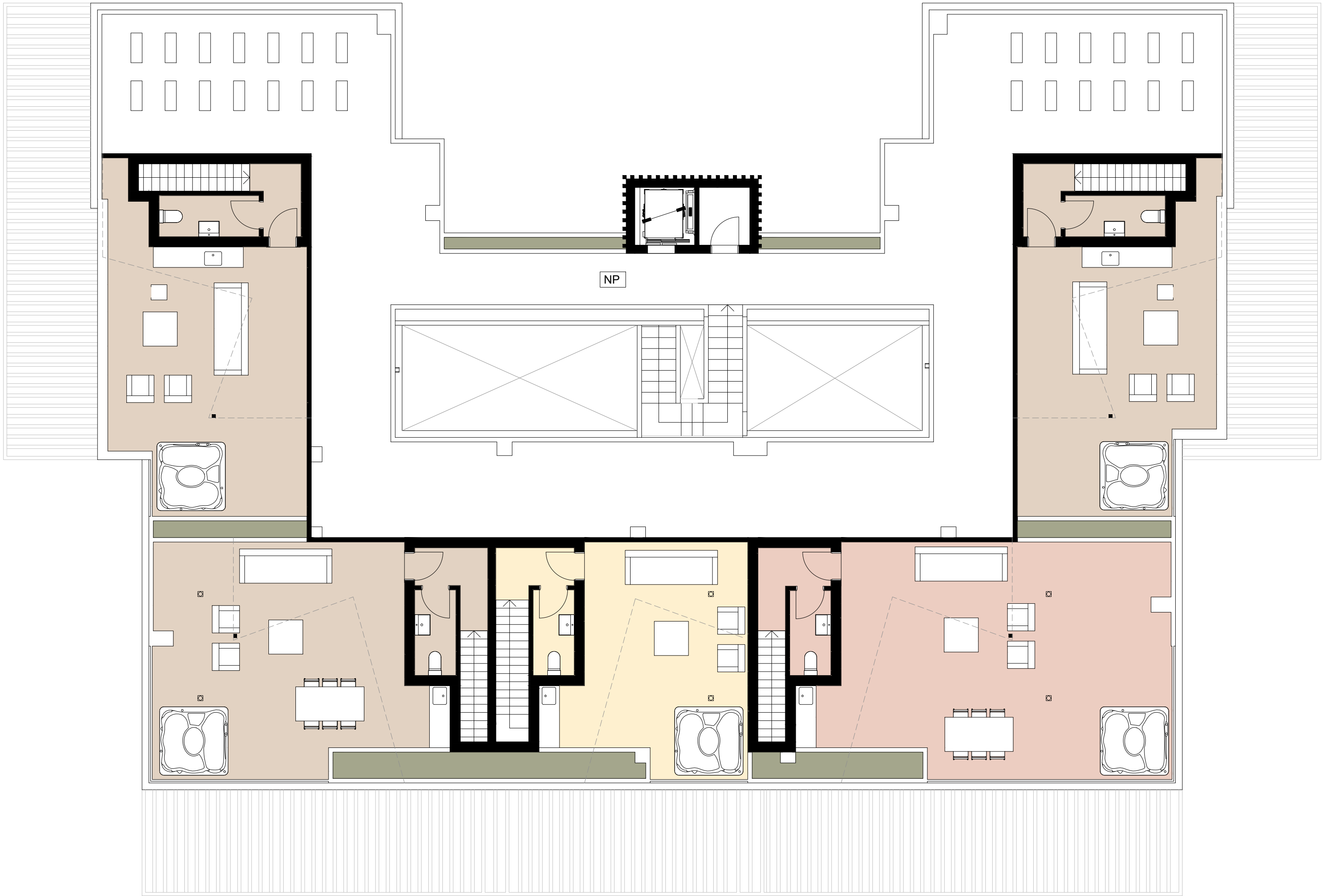
NIVEL PENTHOUSE ESCALA:1 : 150
