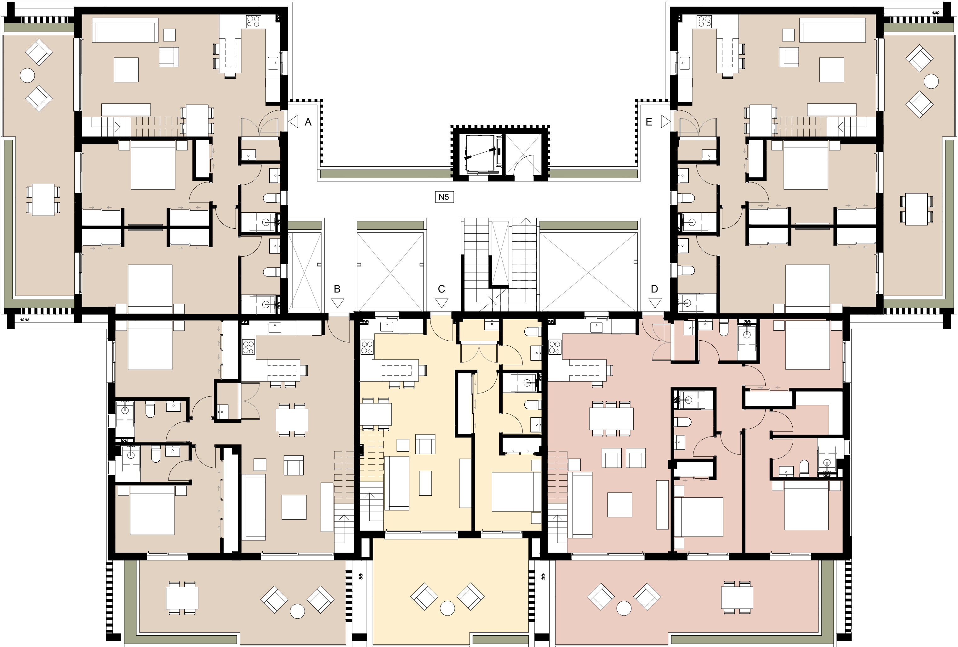
NIVEL 5 ESCALA:1 : 150
