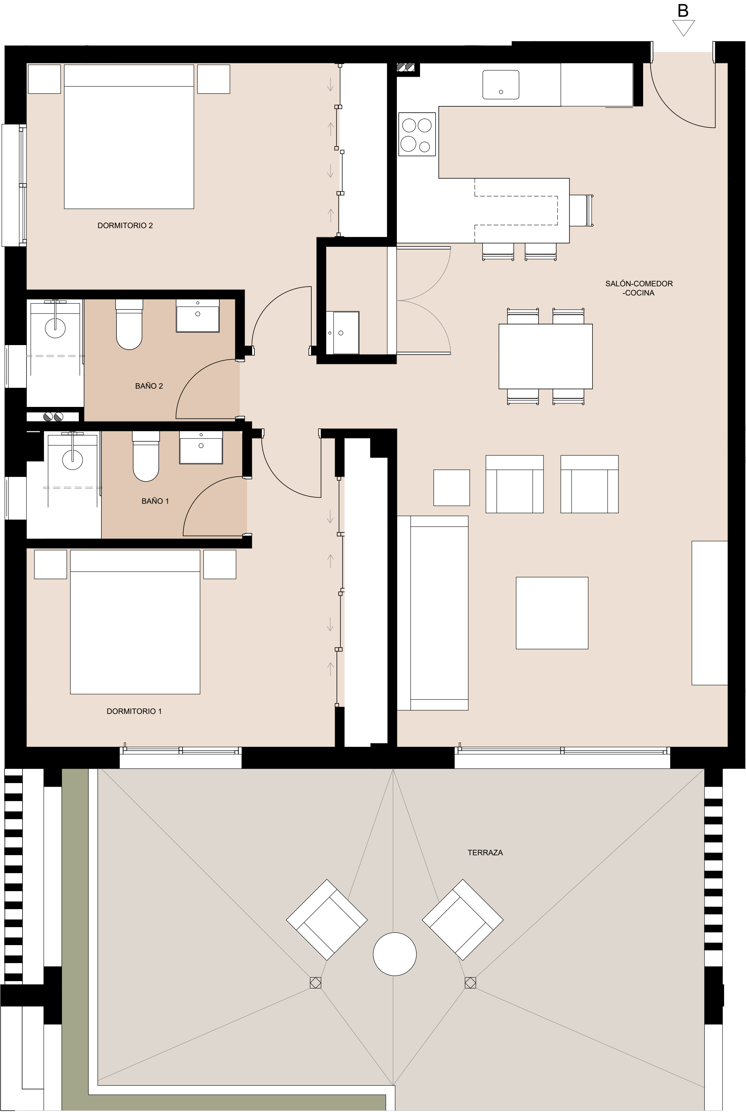
VIVIENDA TIPO B ESCALA: 1 : 50
